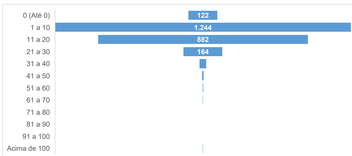
Gráfico 2: Distribuição das ligações residenciais por faixa de consumo (m³/mês)
